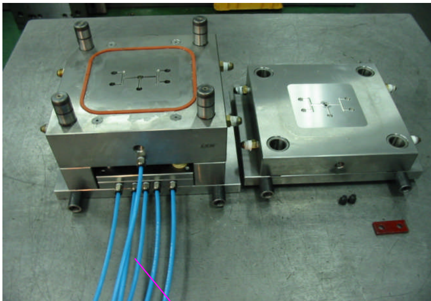
実験金型
